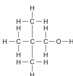
2,2-dimetilpropan-1-ol
